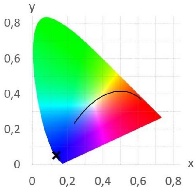
CIE1931:
